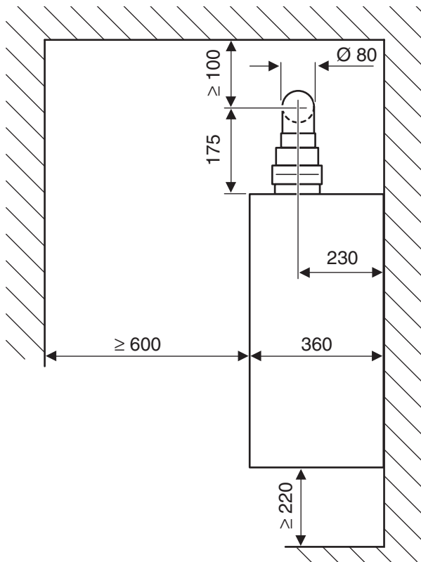
Obr. 10 Odvod spalin v provedení C 42 a C 52
